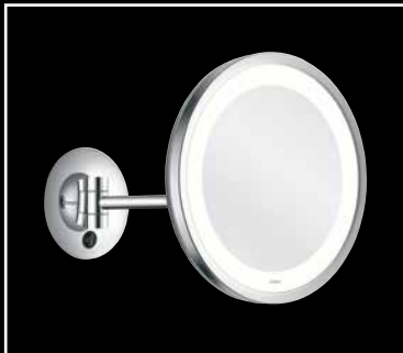
020677 LED CITY LIGHT ø 250 mm. Ausgestreckt 300 mm ø 250 mm. Extends to 300 mm
